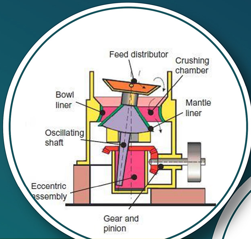
تمصویر ۱ - آسیاب مخروطی یا CONE CRUSHER
