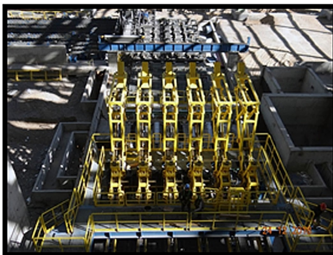
نصب تجهیزات خط ریخته‌گری مداوم
