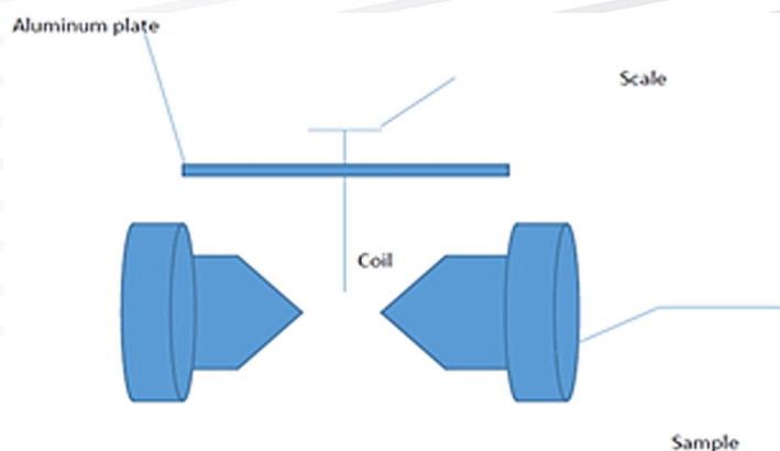
شکل-۱ نمایش از دو آهن ربای الکتریکی که در وسط آن یک میدان مغناطیسی ثابت رو به پایین وجود دارد.
