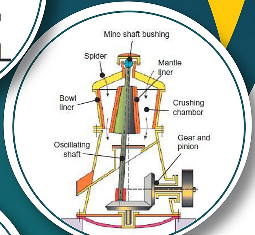
تمصویر ۲ - آسیاب ژیراتوری یا GYRATORY CRUSHER
