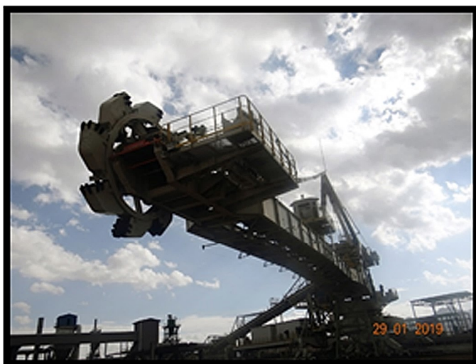
استکر و ریکلایمر ناحیه احیای مستقیم
